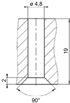
DPG mit Halterung Maximale Schraubenlänge: 19 mm + Stärke der Tischplatte
