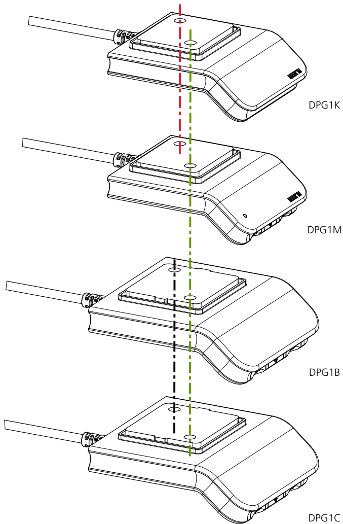
Abbildung 4: Gemeinsame Montagelöcher der verschiedenen DPGs
