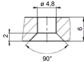
DPG ohne Halterung Maximale Schraubenlänge: 6 mm + Stärke der Tischplatte
